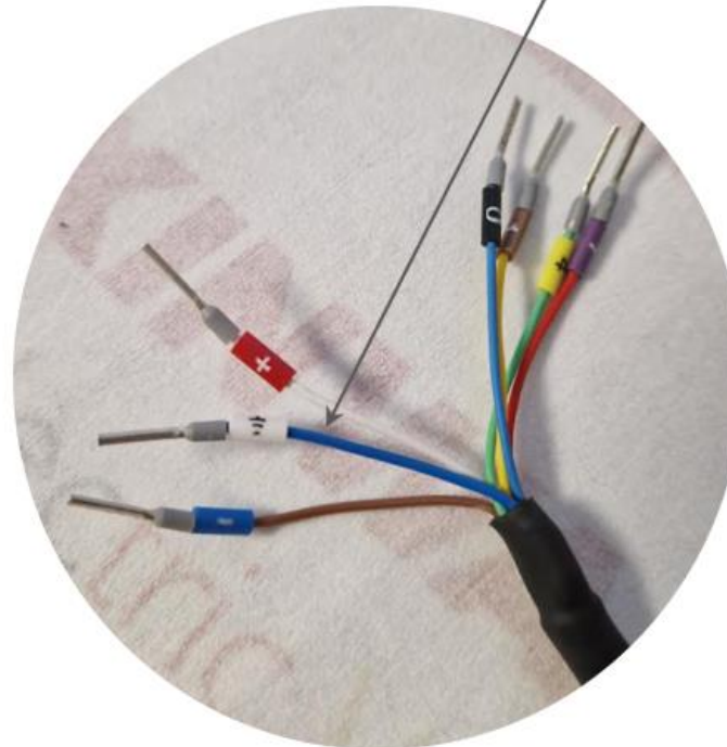
Schirmanschluss
