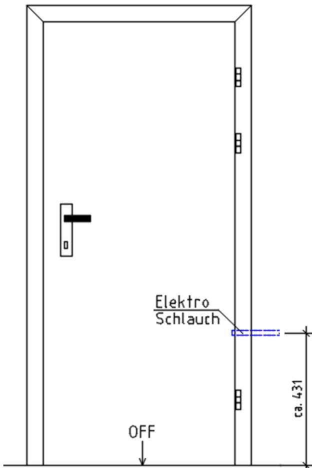
Ausführung gefälzt mit Kabelübergang GU346
