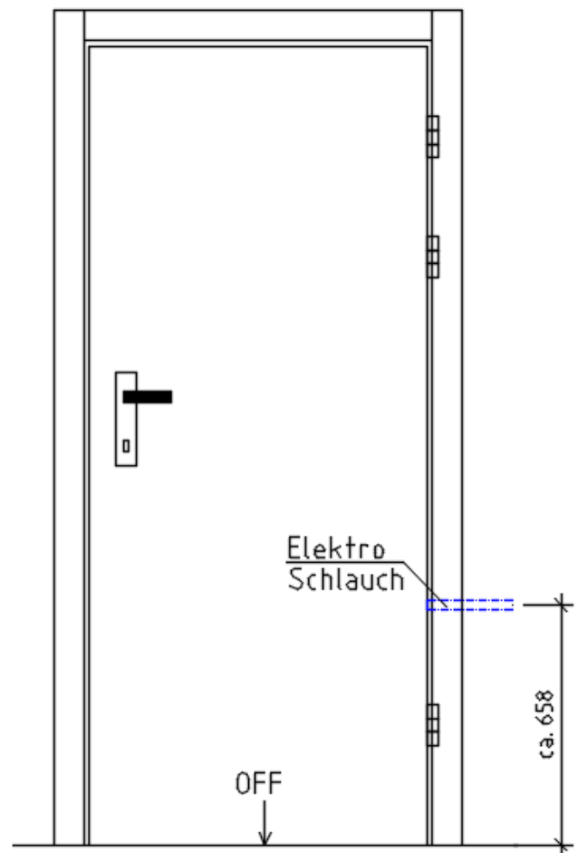
Ausführung Modul mit Kabelübergang eff10314
