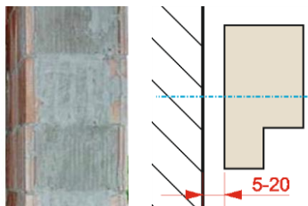
Bild 2: Einbauluft
